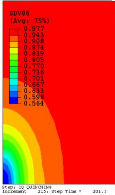
Martensite
