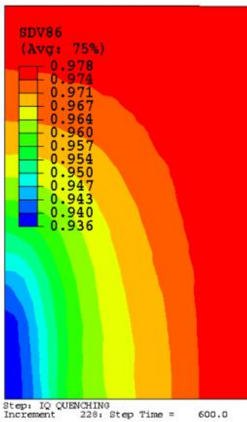
Martensite
